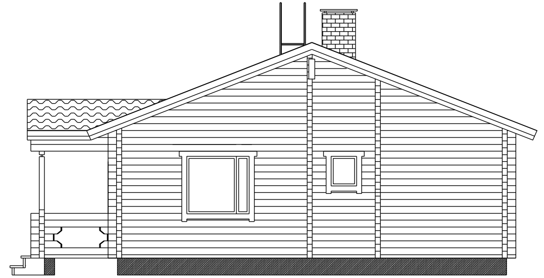
Pääty julkisivu
